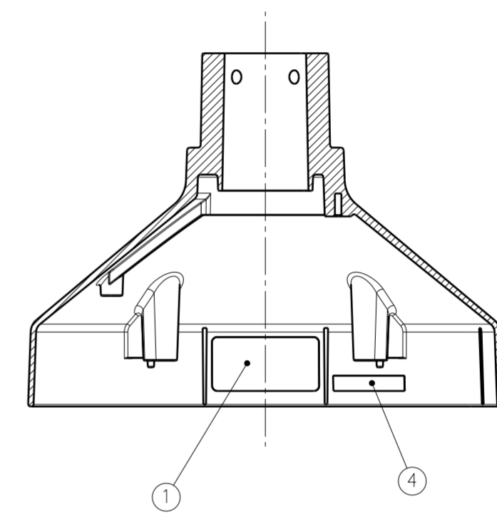
A-A 断面图
