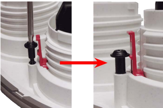
Abb. 18: Sicherungsclip mit Schraube sichern
