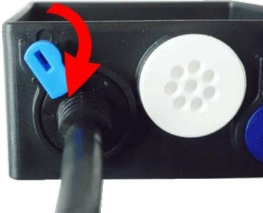
Abb. 26: Stecker des Netzwerkabels in der Anschlussbox verriegeln
